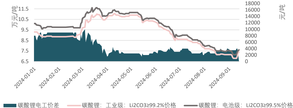
中国碳酸锂现货均价及电工价差
