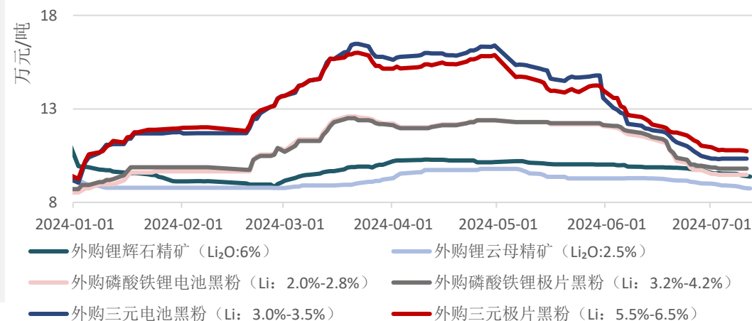
外购原料生产碳酸锂现金成本
